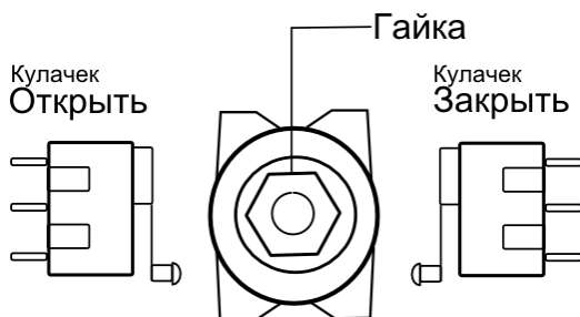
Рис. 86 Настройка концевых выключателей приводов САТУРН ЭП-ЧМ 020-100
