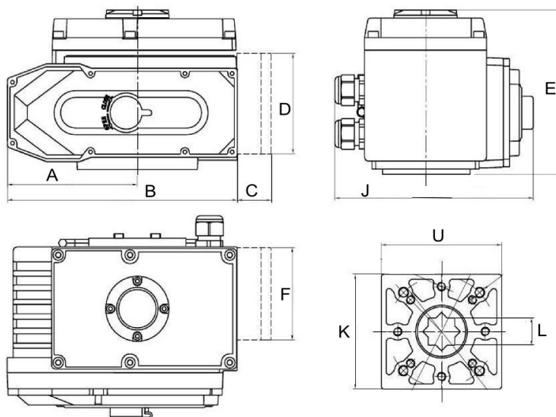
Рис. 3 Габаритные и установочные размеры.
