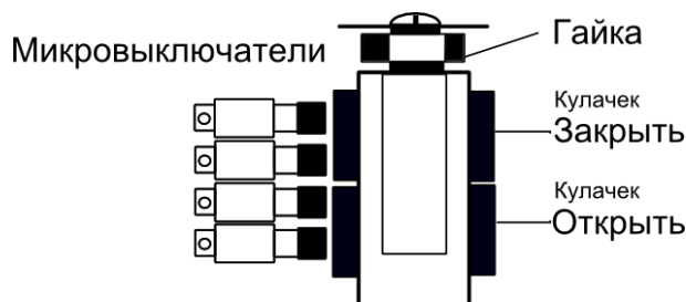
Рис. 8а Настройка конечных выключателей приводов САТУРН ЭП-ЧМ 003-015
